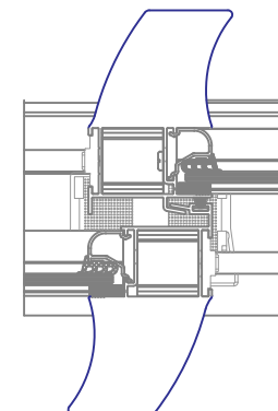
Detalhe de Aplicação Sem Escala
