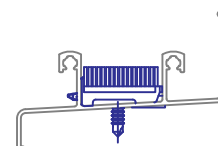
Detalhe de Aplicação Sem Escala
