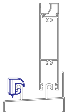
Detalhe de Aplicação Sem Escala
