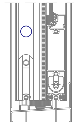
Detalhe de Aplicação Sem Escala
