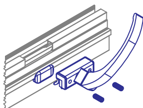
Detalhe de Aplicação Sem Escala
